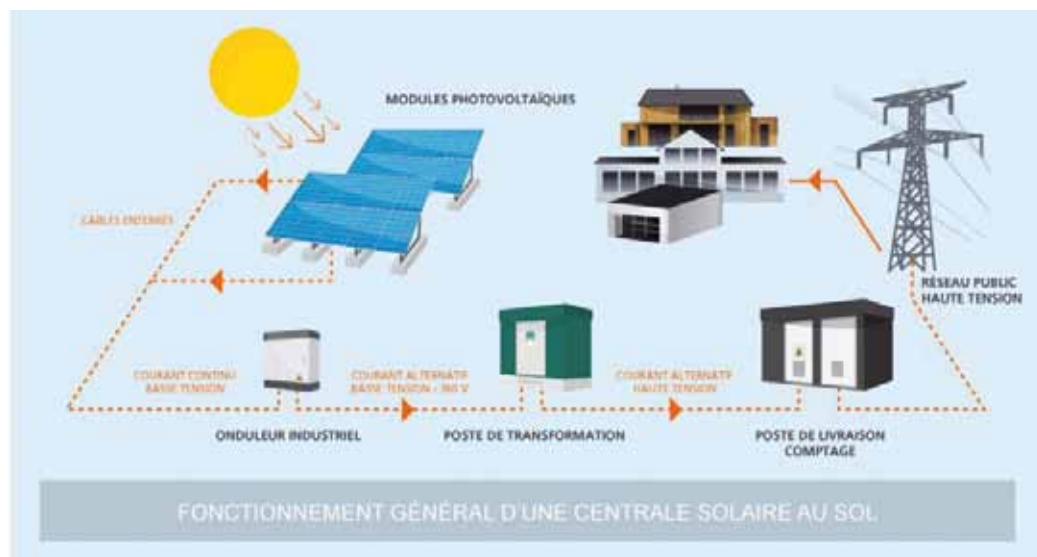
Schéma de principe d'un parc photovoltaïque
